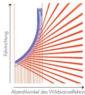
Abstrahlwinkel des Wildwarnreflektors
